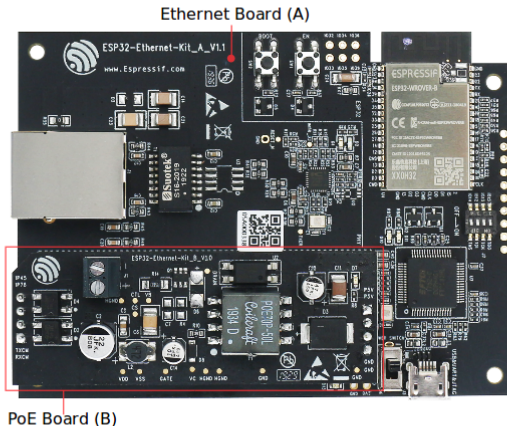
Fig. 12: ESP32-Ethernet-Kit v1.1
