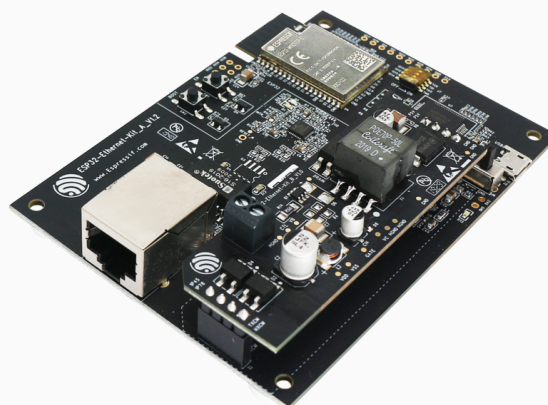
ESP32-Ethernet-Kit
